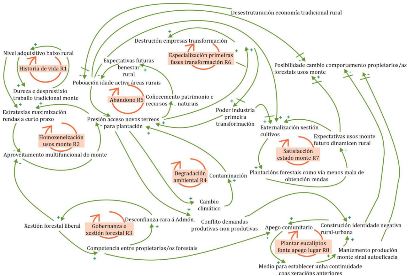
Figura 2. O sistema de retroalimentación entre forestación e abandono do rural. As variables incluídas nos diagramas de bucle (R1-R8) dan conta das conexións e das relacións circulares entre os subsistemas. As malas condicións de vida no rural (R1) favorecen a adopción de estratexias no curto prazo para o aproveitamento do monte (R2). A perda de poboación reduce o coñecemento sobre o terreo e crea unhas expectativas baixas sobre a calidade de vida futura no rural (R5), reforzando a especialización da cadea forestal-madeira nas primeiras fases de transformación (R6). Isto, xunto coa degradación ambiental asociada aos monocultivos e o cambio climático (R4), incrementa a presión polo acceso a novos terreos para as plantacións forestais e coloca nunha situación vantaxosa á industria de primeira transformación de madeira. O sentimento de lugar, composto pola satisfacción respecto da obtención de rendas do monte cun esforzo mínimo (R7) e pola construción dunha identidade rural ancorada no mantemento da súa actividade produtiva e avivada polo conflito das demandas que se lle fan ao monte (R8), crean unha situación na que a probabilidade de acción colectiva é baixa. Un modelo de xestión forestal deficiente incentiva a competencia entre persoas propietarias e a desconfianza entre elas e cara á Administración (R3). Con todo, as posibilidades de que haxa cambios de uso do monte a nivel agregado vense limitadas. Fonte: elaboración propia.
