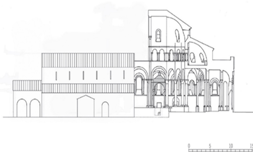
Fig. 4. Corte longitudinal de la catedral de Santiago hacia el año 1105 (J. L. Senra)
