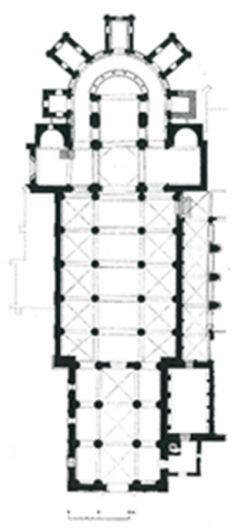
Fig. 11. Planta de la iglesia monástica de Saint-Philibert de Tournus (J. Henriet)
