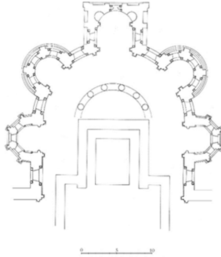
Fig. 3. Planta hipotética de la cabecera de la catedral de Santiago hacia el año 1095 (J. L. Senra)
