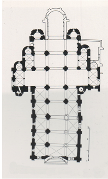
Fig. 8. Planta de la iglesia monástica de Saint-Sever (J. Cabanot)
