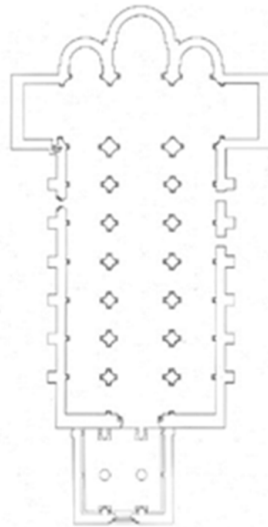
Fig. 6. Planta hipotética de la iglesia románica de Sahagún con añadido de bloque occidental (J. L. Senra)
