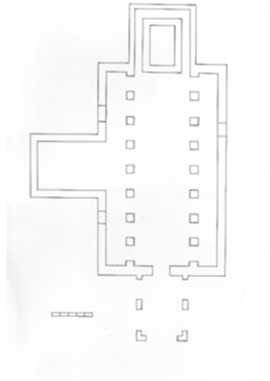
Fig. 1. Planta iglesia de Santiago financiada por Alfonso III (J. Guerra Campos)
